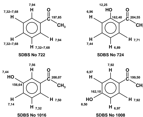
Рис. 2. Некоторые 1 H и 13 C ЯМР-сигналы в спектрах ацетофенона и его орто-, мета- и пара-гидроксипроизводных по данным сетевой базы SDBS [27]
